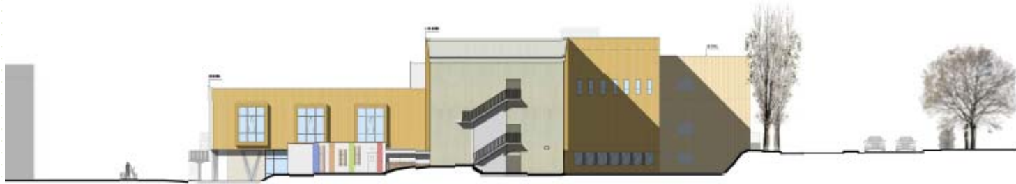
FACADE EST échelle 1/200 eme
